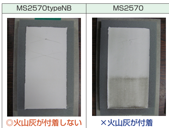
■ アクリル樹脂エマルジョン塗料の塗料付着性・汚染性試験例
